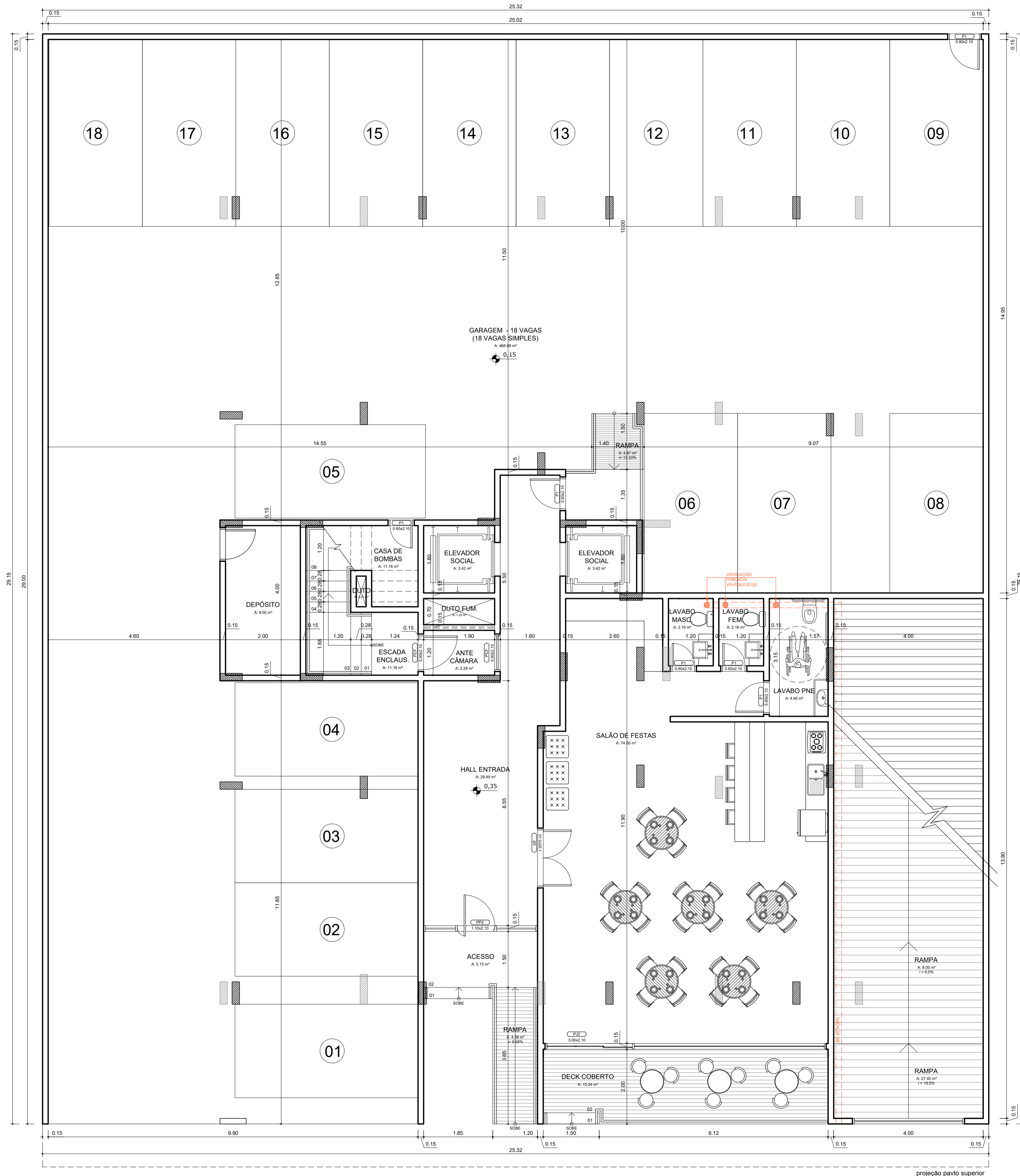
PLANTA BAIXA PAVTO TÉRREO - TORRE 01/ 02/ 07/ 08/ 09 ÁREA DO PAVTO: 738,12 m 2 ÁREA COMPUTADA: 605,82 m 2
